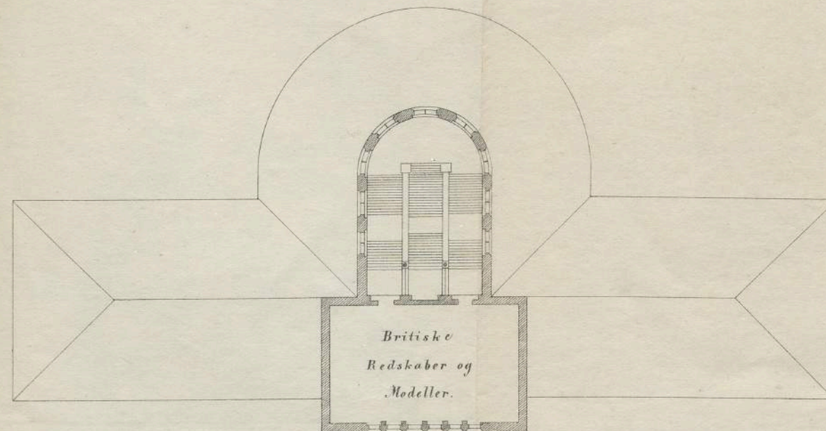
Grundrids af 3 ste Etage
